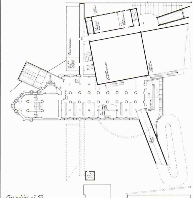
Grundriss -1.50
