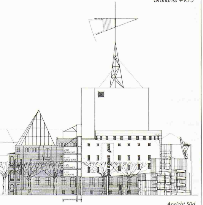
Ansicht Süd
