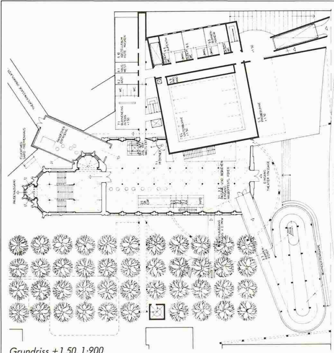
Grundriss +1.50, 1:900
