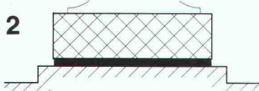
Maschinensockelisolierung
