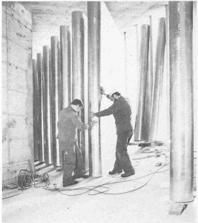
Bild 5. Montage der Kulissen-Schalldämpfer beim Abluftbauwerk Rütelen
