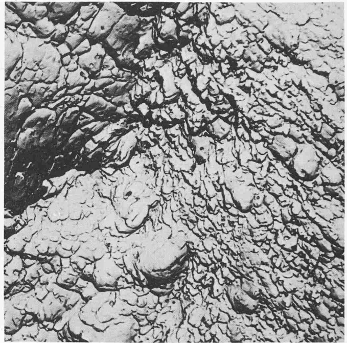
Gewaltbruchfläche an Konstruktionsteil, elektronenoptisch dargestellt
