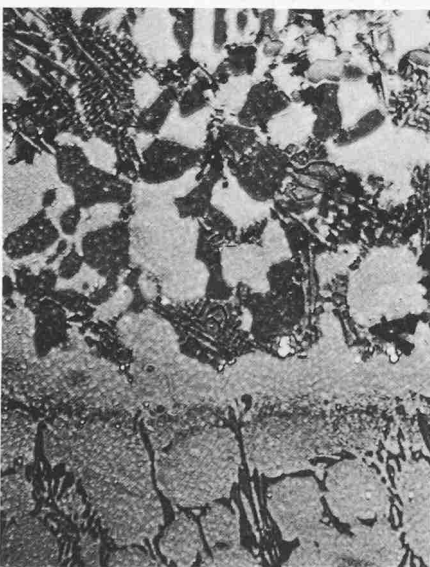
Dieselmotorauspuffventil mit gepanzelter Sitzfläche: Auf die Stelliteunterlage (Kobaltbasis mit Chrom-Wolfram-Karbid-Netzwerk) ist eine Superlegierung als Korrosionsschutzschicht (oben) aufgespritzt. Um das Mikrogefüge im Farbkontrast sichtbar zu machen, wurde die Verbindungzone im Vakuum mit Zinkselenid bedampft
