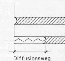
Bild 1. Oben: Wasserfaden in der Kapillare bis an die Oberfläche vorgezogen. Unten: Verdunstung ist stärker als der kapillare Nachzug, längerer Diffusionsweg
