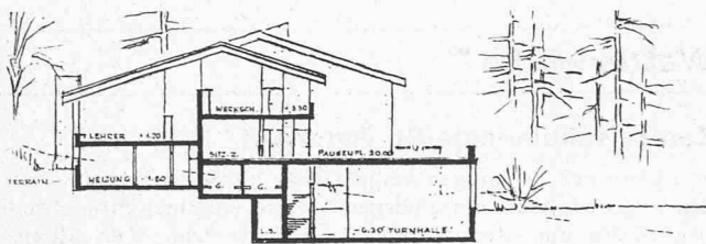
Schnitt Lehrerzimmer-Turnhalle 1:600
