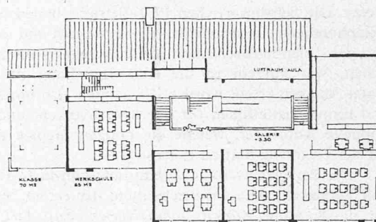
Grundriss Galeriegeschoss 1:600
