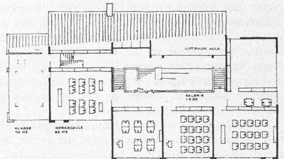
Grundriss Galeriegeschoss 1:600
