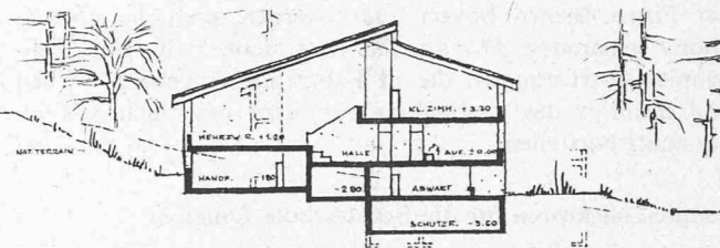
Schnitt Mehrzweckraum-Abwart 1:600
