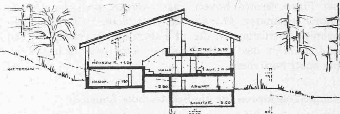
Schnitt Mehrzweckraum-Abwart 1:600
