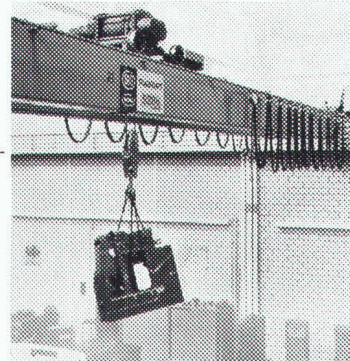
SIG-KULI-Zweiträger-Laufkran
