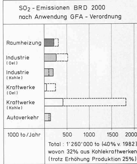
Bild 3. Schwefeldioxid-Emissionen im Jahr 2000 in der Bundesrepublik Deutschland nach Anwendung der Grossfeuerungsanlagen-Verordnung. Vergleichswerte 1982. Quelle: Brennstoff-Wärme-Kraft, H. 10, Okt. 1983
