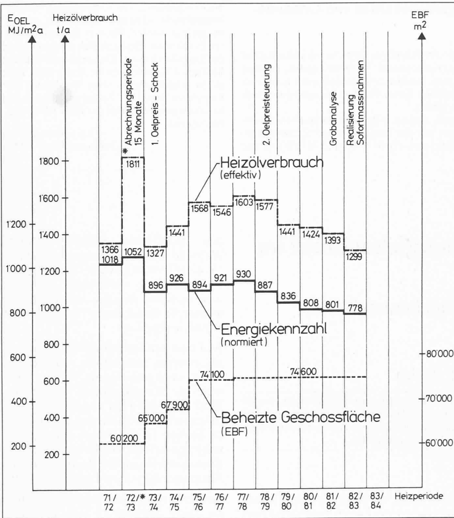
Bild 1. Entwicklung der beheizten Geschossfläche, des effektiv abgerechneten Heizölverbrauches und der normierten Energiekennzahl (E Oel ) für einen Gebäudebestand von 34 Liegenschaften mit total 97 Mehrfamilienhäusern (Stand 1983)
