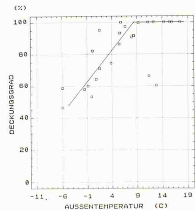
Anteil Waermelieferung der WP am Gesamtwaermebedarf, Messdaten 1984-1987
