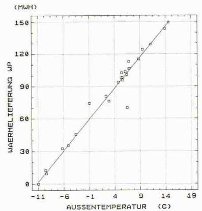
Waermelieferung und Primärenergieverbrauch der Wärmepumpe, Messdaten 1984-1987
