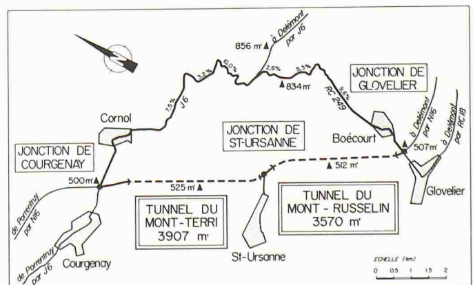
Situation des quatre portails de tunnel
