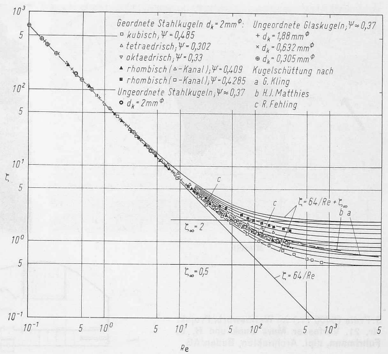
Bild 20. Widerstandszahl \zeta nach Gl. (23) in Abhängigkeit von Re = wd/v
