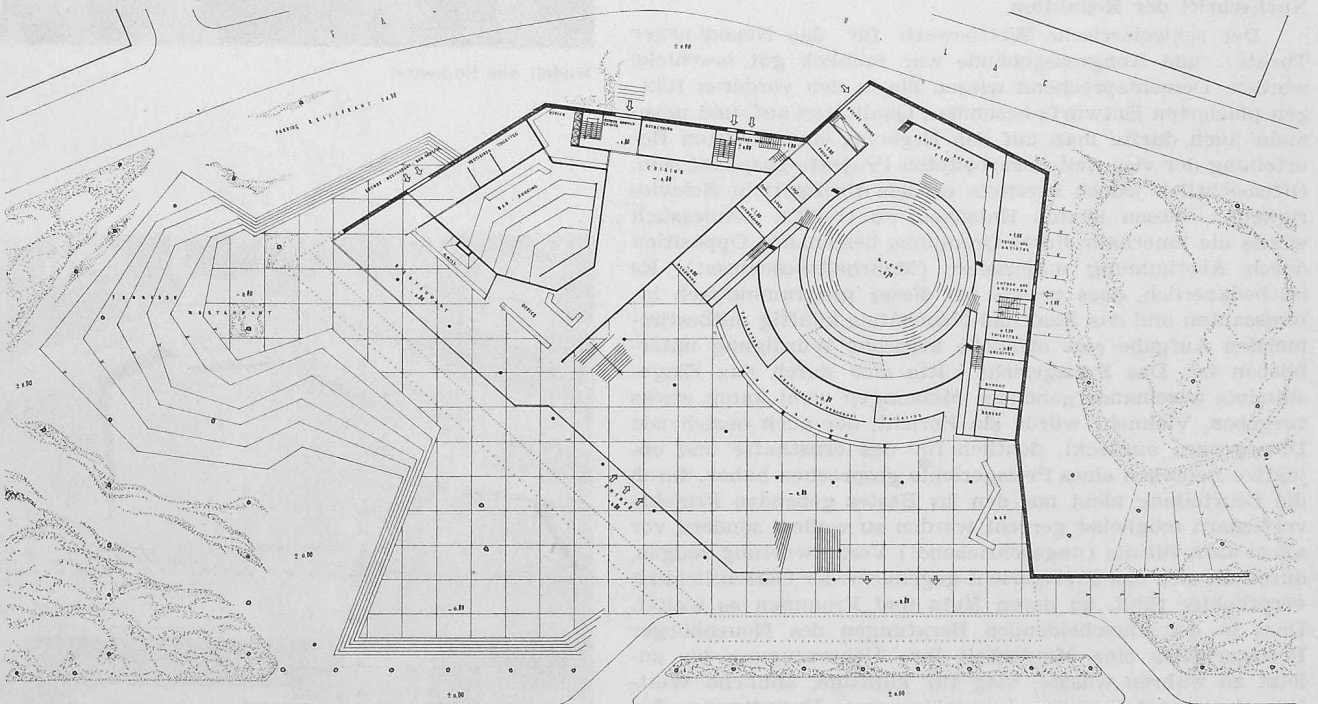
Eingangsgeschoss, 1:900
