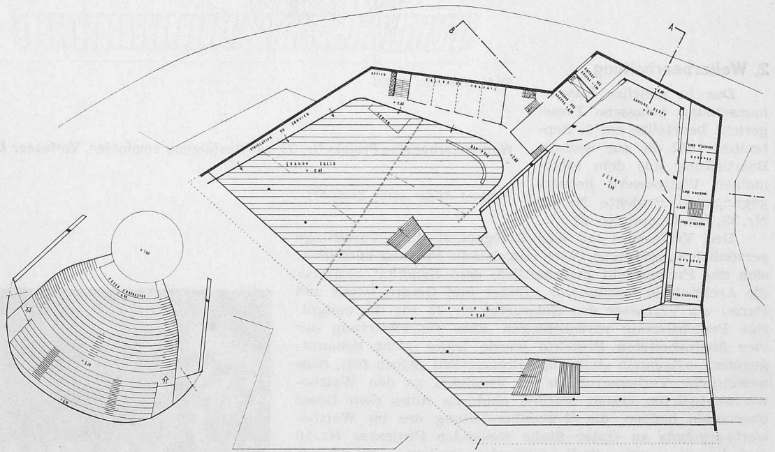
Obergeschoss-Grundriss, 1:900
