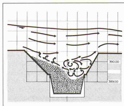
Bild 4. Ohne Traverse bildet sich eine pulsierende Strömung, einzelne Wirbel und Wasserwalzen wirken zu stark nach der Tiefe und verhindern das angestrebte Absetzen von Steinen
