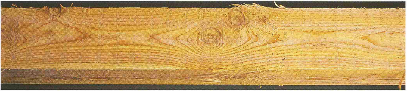
Bilder 2a, 2b, 2c. Störung des Faserverlaufs bzw. der Holzstruktur durch Äste. Die Aststörzone kann um ein Vielfaches grösser sein als der eigentliche Ast.
