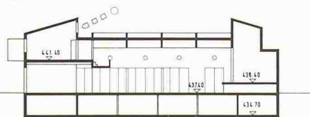
Schnitt Saal
