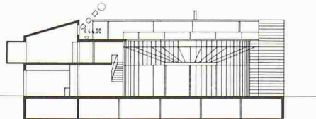
Schnitt Hof
