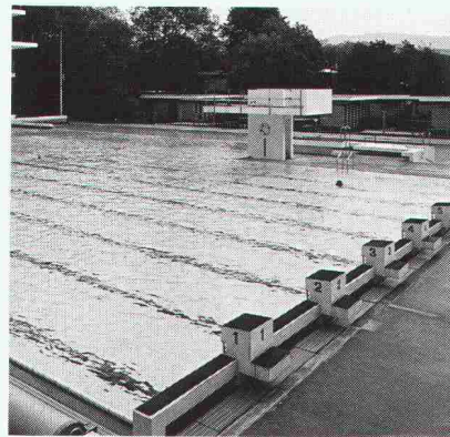
Basel Sportbad St. Jakob: Wasserverluste durch undichte Fugen verlangen eine sofortige Sanierung. Gezielte Injektionen machen das Bassin wieder dicht.
