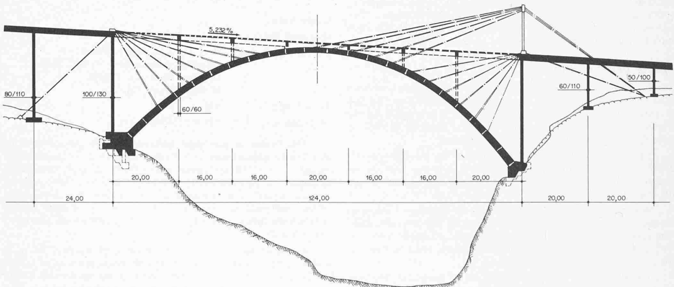
Bild 11. Krummbachbrücke. Freivorbau des Bogens mit Hilfe der Rückhalte cables Krummbachbrücke. Cantilevering-out of the arch with the aid of the tie-back cables
