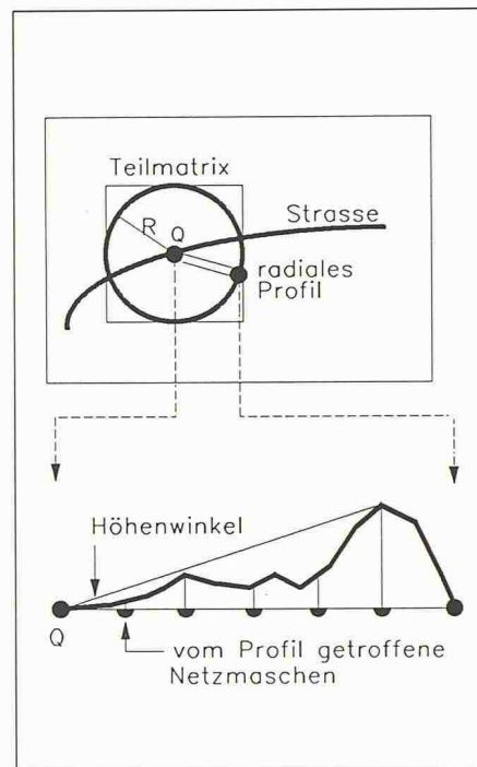
Bild 3. Funktionsweise des Algorithmus zur Ausbreitungsrechnung ( Q = Quellmasche, R = wählbare maximale Ausbreitungsdistanz)
