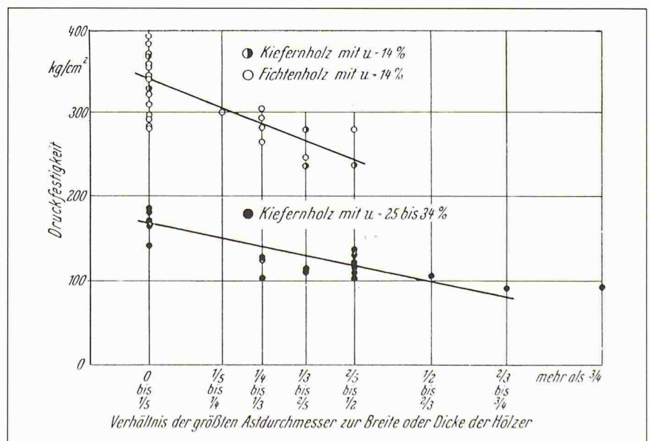
Bild 3. Druckfestigkeit von Fichten- und Kieferholz in Abhängigkeit von der Astgrösse (nach Graf [1938])
