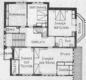
Abb. 10 u. 11. Grundrisse vom Erdgeschoss und ersten Obergeschoss der Villa «Hadlaub» in Zürich IV. — 1 : 400. Erbaut von Pflughard & Haefeli, Architekten in Zürich.
