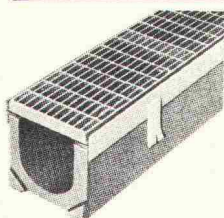
FASERFIX-Rinne mit T-Profil und Gitterrost (10 t RD)
