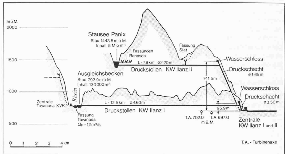
Bild 2. Längenprofil
