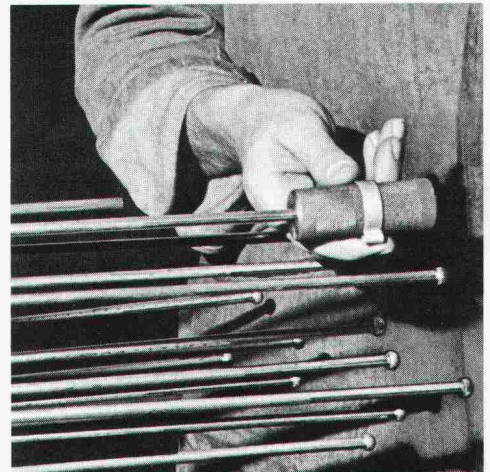
Kontrolle der Abmessungen von BBRV-Stauchköpfen
