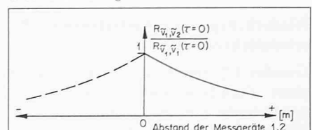
Bild 5b. Genereller Verlauf der Kreuzkorrelation in Funktion des Signalabstandes
