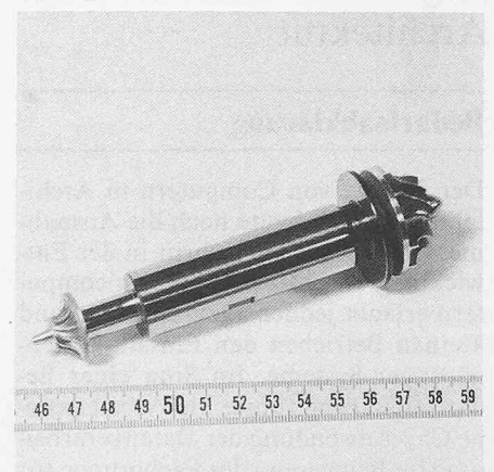
Rotor einer Heliumturbine (Drehzahl bis 300 000 U/min); links der Expanderrotor, rechts der Bremskompressor
