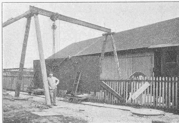
Abb. 12. Transporeinrichtung für die Blechtafeln.
