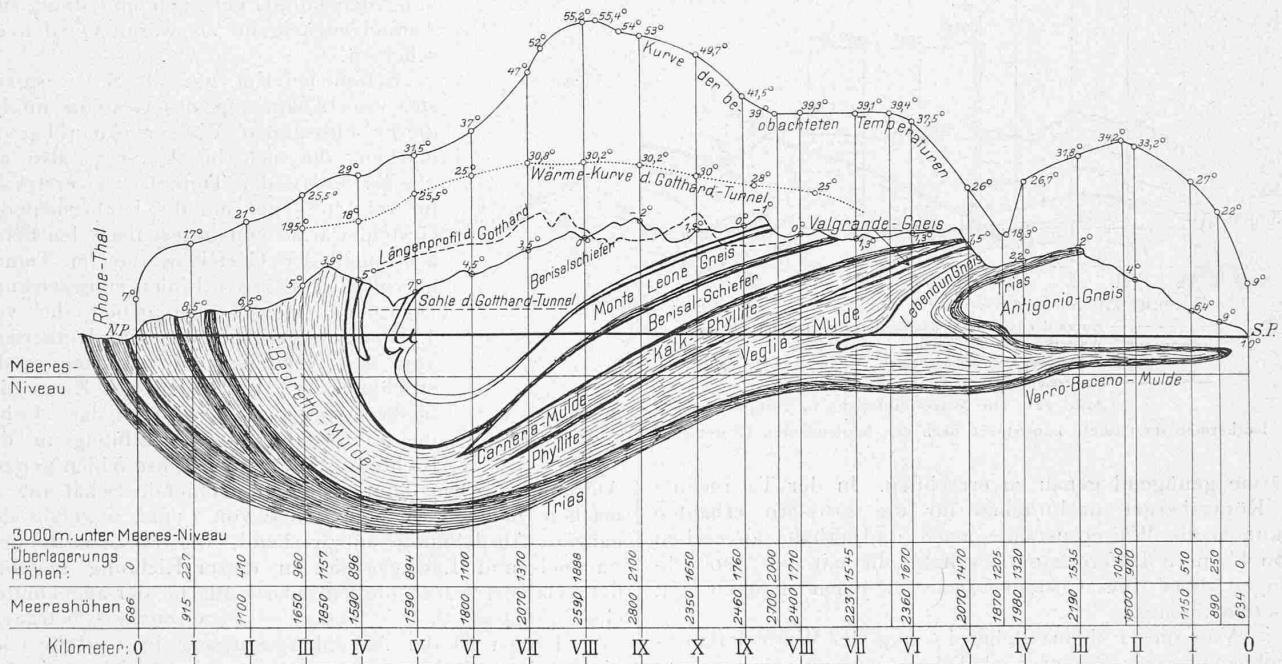
Abb. 21. Profil längs der Achse des Simplontunnels (Einpunktigt Gotthardtunnel) und geologisches Profil. — 1 : 120 000.
