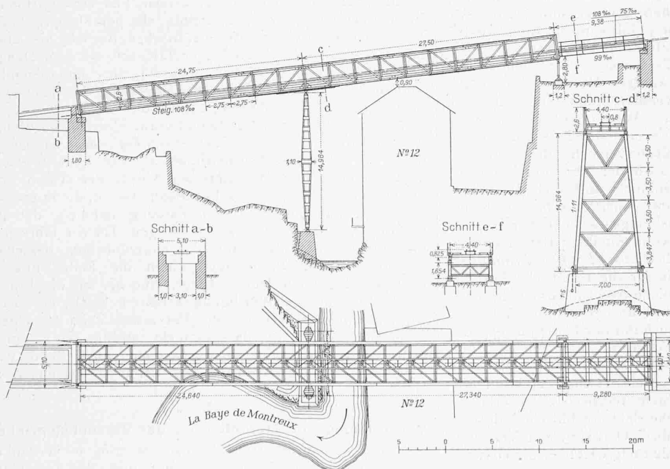
Abb. 26. Eiserner Brücke über die Chauderon-Schlucht. — Masstab 1 : 500.
