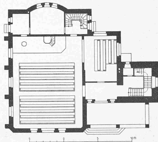
Abb. 2. Grundriss. — 1:300.
