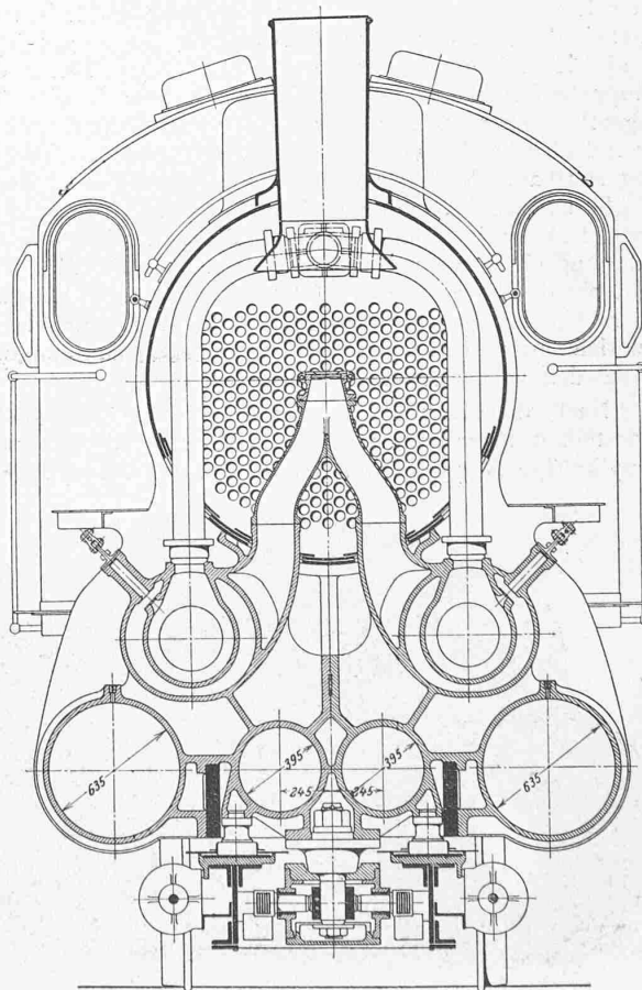
Abb. 6. Schnitt durch die Rauchkammer. — 1:35.
