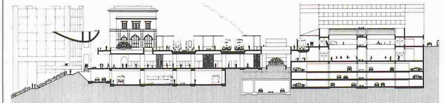
Sezione trasversale
