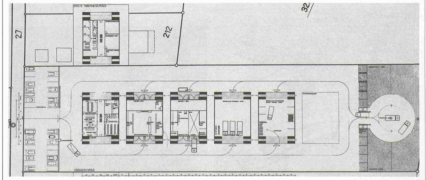
Grundriss Erdgeschoss
