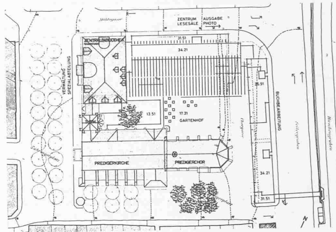
Lageplan 1:1700
