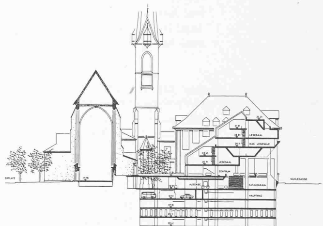
Schnitt Predigerplatz-Mühlegasse 1:1100 Ansicht von Norden 1:1100
