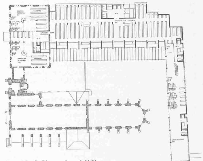
Grundriss 3. Obergeschoss 1:1100
