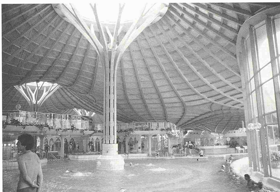
Bild 5. Höhepunkt des Holzbaus ist die vollkommene Synthese der Funktionen «Tragen», «Raumtrennen» und «Gestalten». Bild: Holzrippenschale der Dachkonstruktion des Solebades in Bad Dürrenheim
