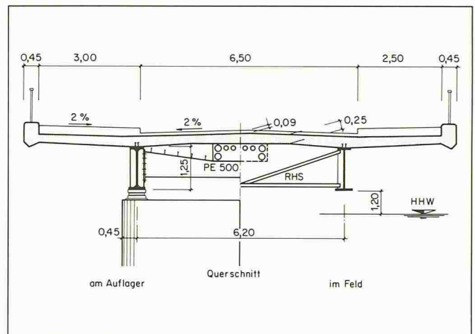
Bild 3. Brückenquerschnitt
