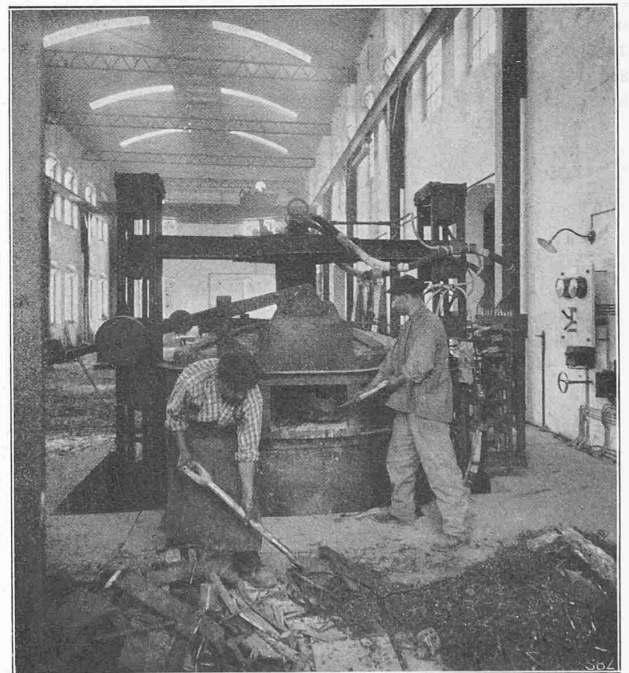
Abb. 2. Chargierseite; Einsatzmaterial.
