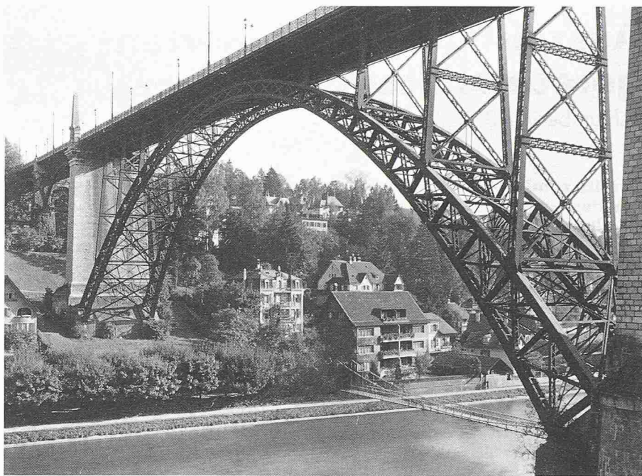
Die Kornhausbrücke in Bern, erbaut 1895–1898, Stahlgewicht 1815 t
