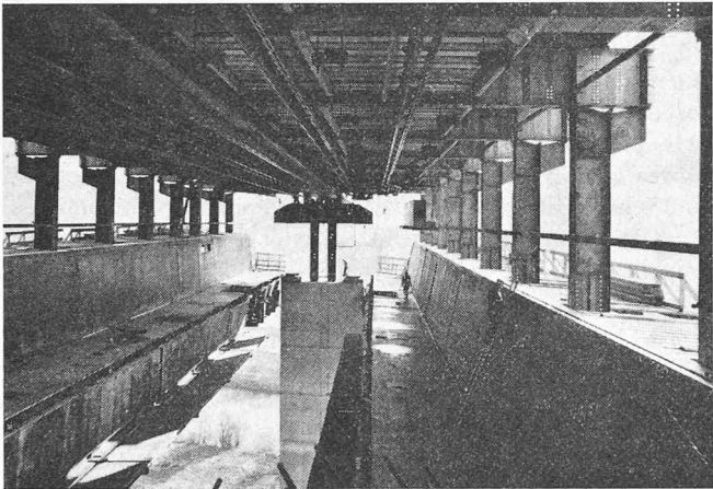
Bild 7. Das Gerüst steht kurz vor der Vollendung der Vorfahrt ins neue Feld. Das Stützenpaar auf dem freien Pfeiler wurde aus der vorhergehenden Stellung am Vorbauschnabel hängend in die hier gezeigte Stellung verschoben, um den neuen, vordern Stützpunkt zu bilden. Der Trogboden ist zum Teil nach unten geklappt, die ganze Schalung in zwei Hälften je seitlich ausgeschoben, um die Vorbeifahrt am Pfeiler zu gestatten.
