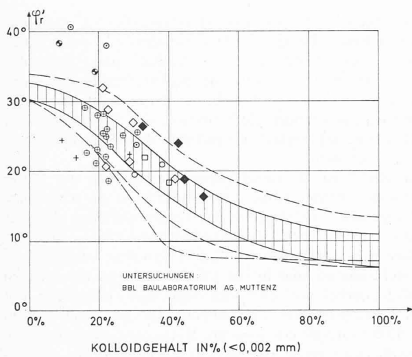
Bild 8. Scherwinkel in Abhängigkeit des Kolloidgehaltes für Proben der Juraformation
