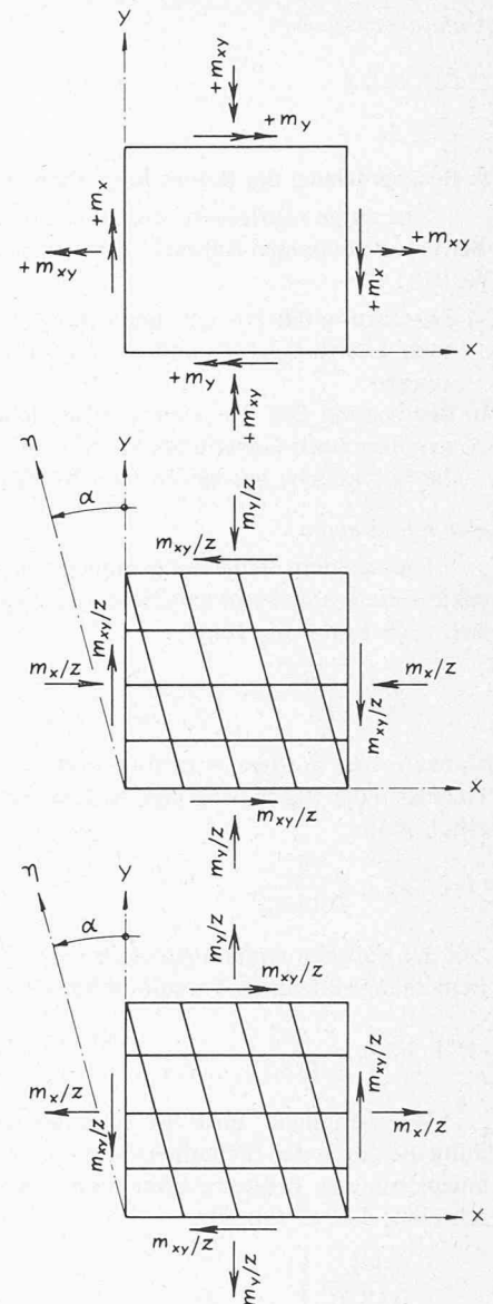
Bild 5. Wirkung der Plattenmomente. Oben: Draufsicht Mitte: Oberseite Unten: Unterseite
