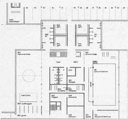
Kantinentrakt Untergeschoss 1:900
