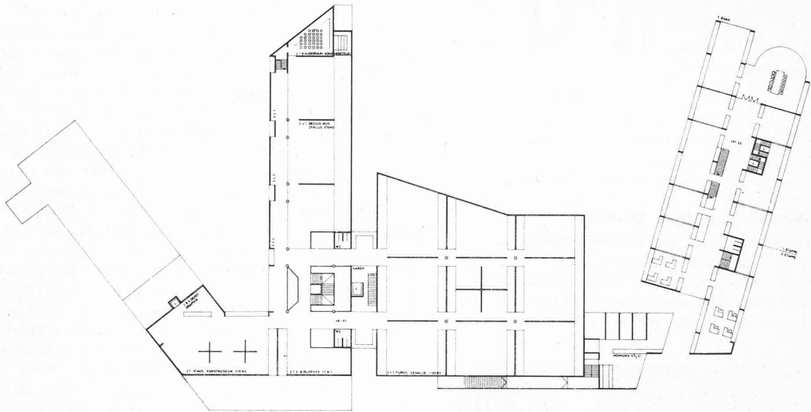
Grundriss 1. Obergeschoss 1:900
