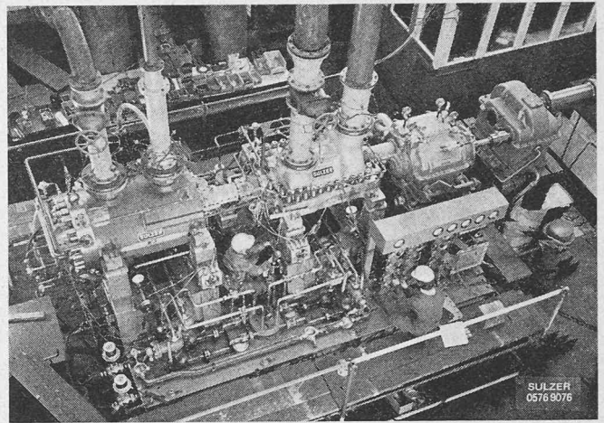
Einer der drei Turbokompressoren für die Sasanfield-Plattform während der Probeläufe im Werk
