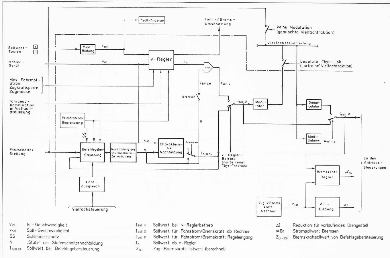
Bild 28. Loksteuerung, Blockschemata
