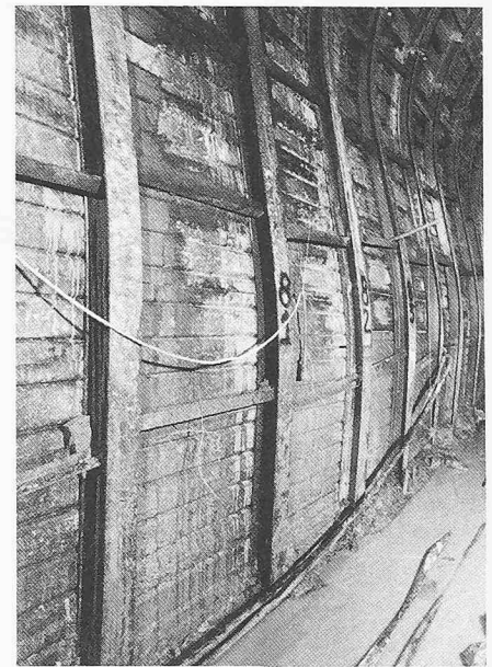
Bild 7 (oben). Hufeisenprofil. Deformationen im Stahlbau bei Tm 8500
