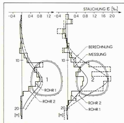
Bild 3. Gestaffelter Vortrieb zweier Tunnelröhren: Vergleich des gemessenen und berechneten Verlaufes der Stauungen im Baugrund (Kovari/Amstad)
