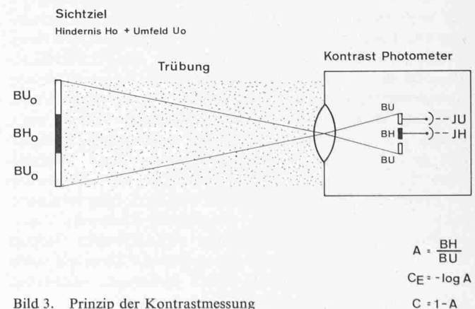
Bild 3. Prinzip der Kontrastmessung
