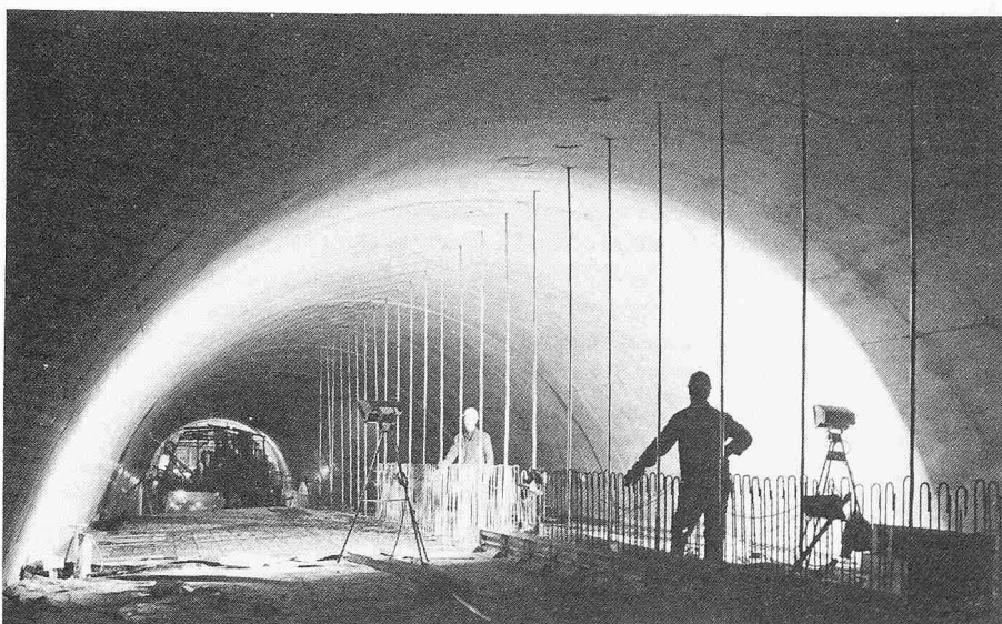
Bild 18. Einschalen der Zwischendecke für die Lüftungskanäle über dem Fahrraum (Abb. 12)
