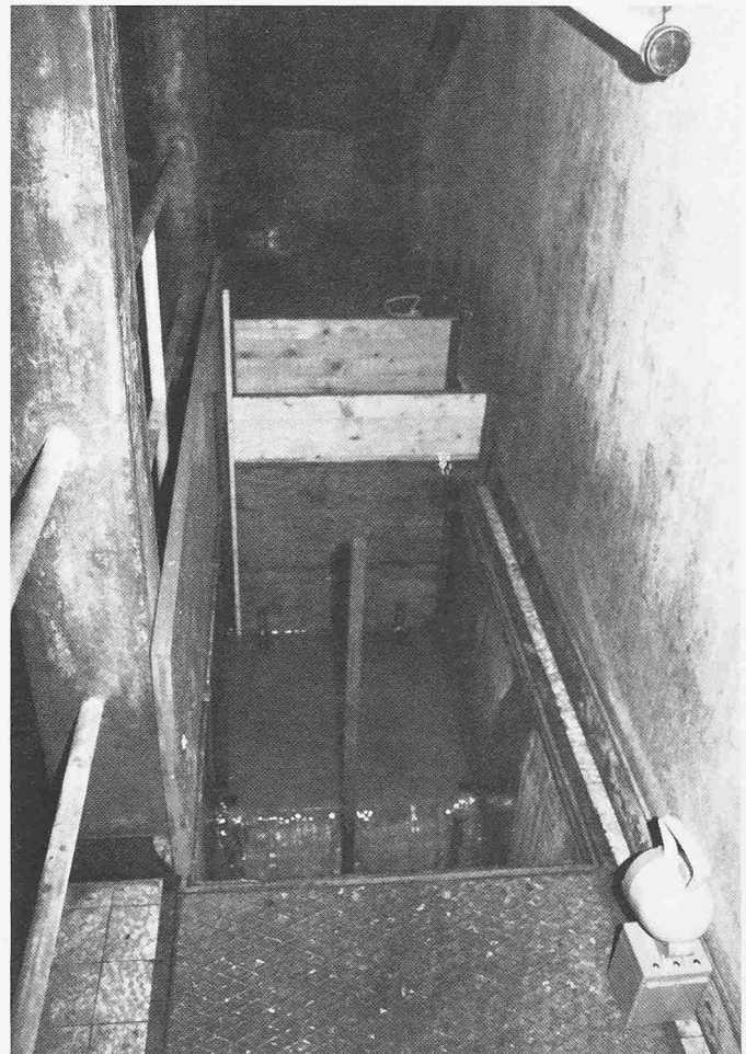
Bild 2. Versuchsanordnung: Versuch im Gang. Ein Foto, das den Kanal während des Versuchs zeigt. Wasser strömt von unten nach oben durch das Sieb. Die Siebfläche ist mit Schmutzpartikeln bedeckt. Die Holzstützen sind ebenfalls sichtbar.
