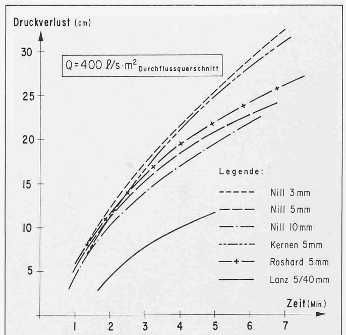
Bild 11. Druckverlust der untersuchten Siebe für eine spezifische Siebbelastung von 400 \text{ l/s} \cdot \text{m}^2 freier Durchflussquerschnitt, für rohes unverdünntes Abwasser
