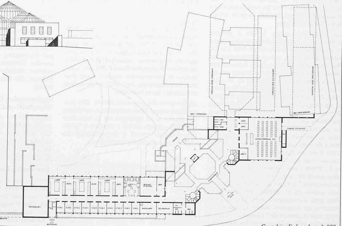
Grundriss Erdgeschoss 1:800
